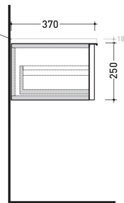
sezione longitudinale / section
